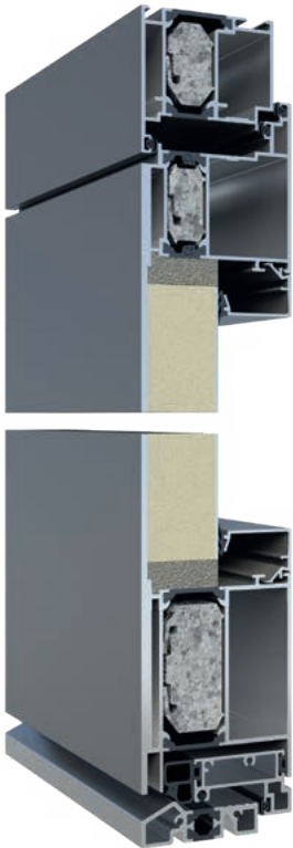
Abb. flügelüberdeckende Füllung außen (Mehrpreis)
